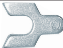
205-005 Calços de Cambagem A,C,D-10 E A,C,D-20 .. /92 1,00mm
