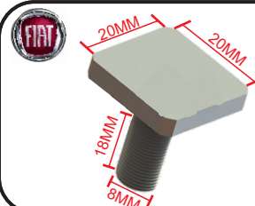
604-007 Grampo Alto Falante Palio Weekend Siena Strada
