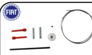
103-504-003 Kit Cabo do Tempra Diant. 93/94 4 Portas
