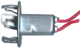
156-307 Soquete garra pinos transversais 2 polos
