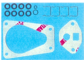
106-230-019 Junta p/ Injeção Elet. Vectra/ Calibra 2.0 16v Sistema Bosch M-28
