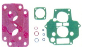
108-201-201 Jogo de Junta Carb. Chevette 1.6 - Mod. 460 - Duplo
